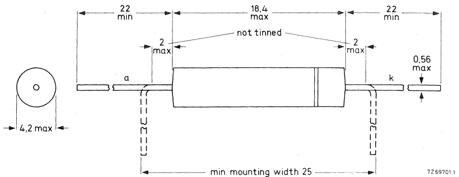
Fig. 1 SOD-56.
