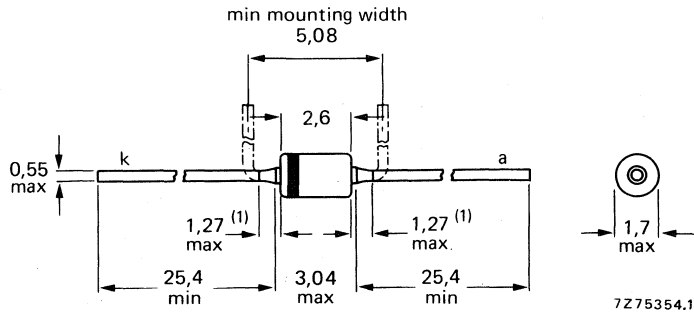
Fig. 1 SOD-58 (DO-34).
