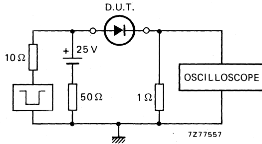
Fig. 6 Test circuit. Input impedance oscilloscope 1 M \Omega ; 22 pF. Rise time \leq 7\text{ ns} . Source impedance 50 \Omega . Rise time \leq 15\text{ ns} .
