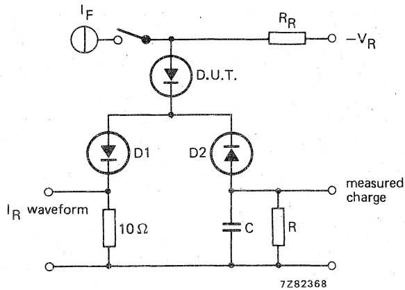
Fig. 2 Test circuit.
