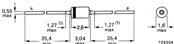
Fig. 1 SOD-68 (DO-34).
