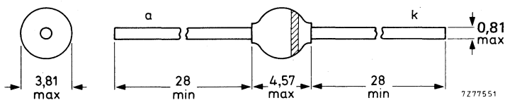
Fig. 1 SOD-57.
