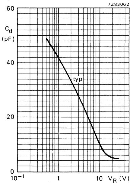
Fig. 4 f = 500\text{ kHz} ; T_{\text{amb}} = 25\text{ }^\circ\text{C} .
