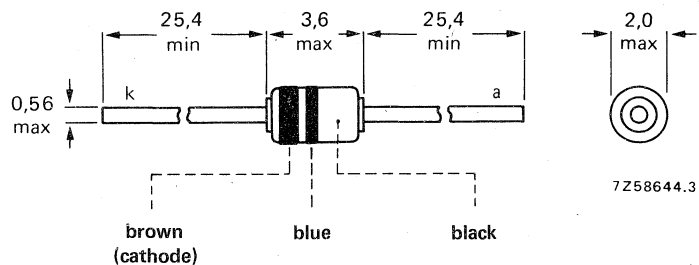
Fig. 1 SOD-17 (DO-35).
