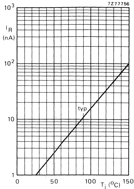
Fig. 3 V_R = 20\text{ V} .
